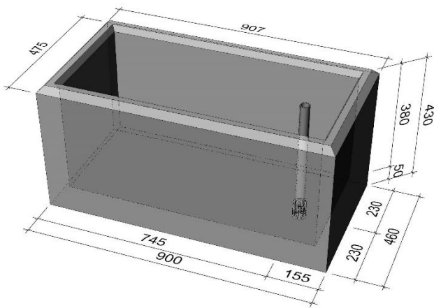
Bemassung
