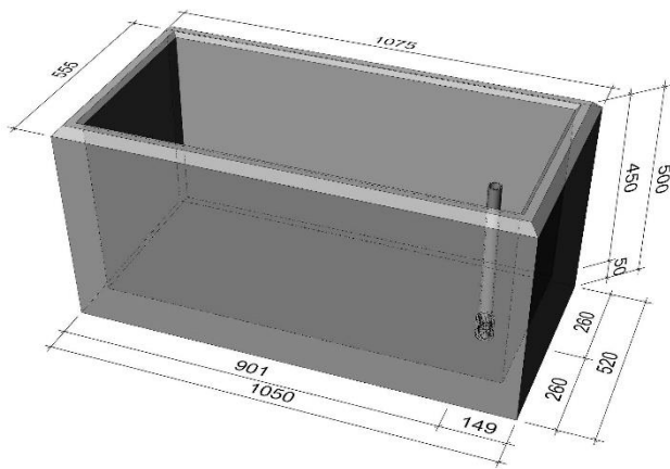
Bemassung
