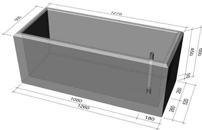
Bemassung
