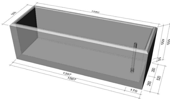
Bemassung
